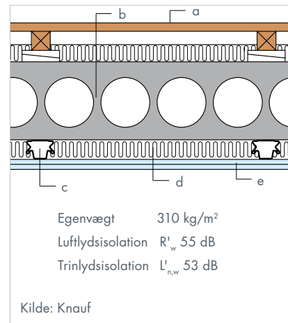
220 mm betonthuldæk med strøgulv
