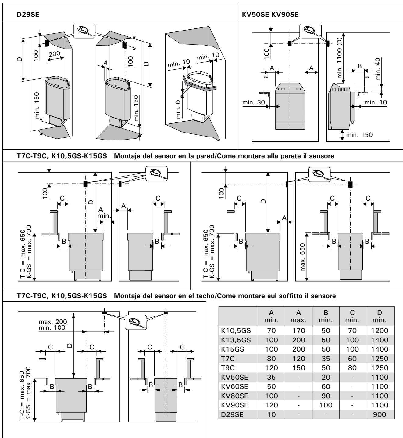
Figura 5. Distancias de seguridad (todas las dimensiones en milímetros)
