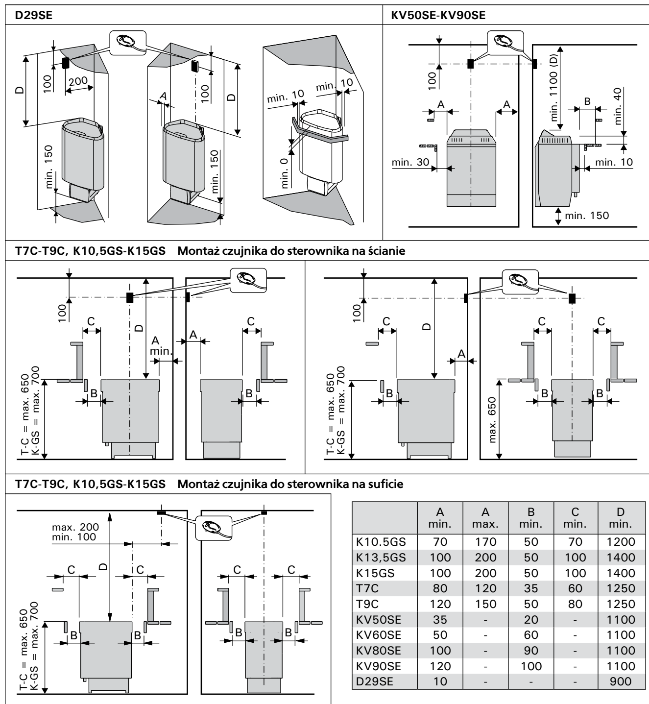
Rys. 5. Minimalne odległości instalacyjne (wymiar w milimetrach)
