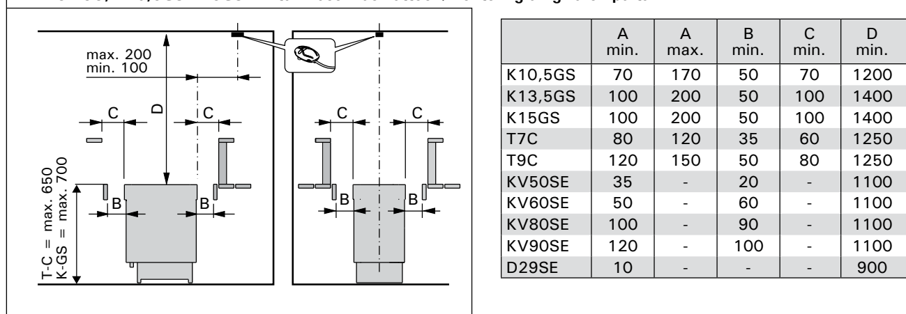
Kuva 5. Kiukaan suojaetäisyydet (mitat millimetreinä)
