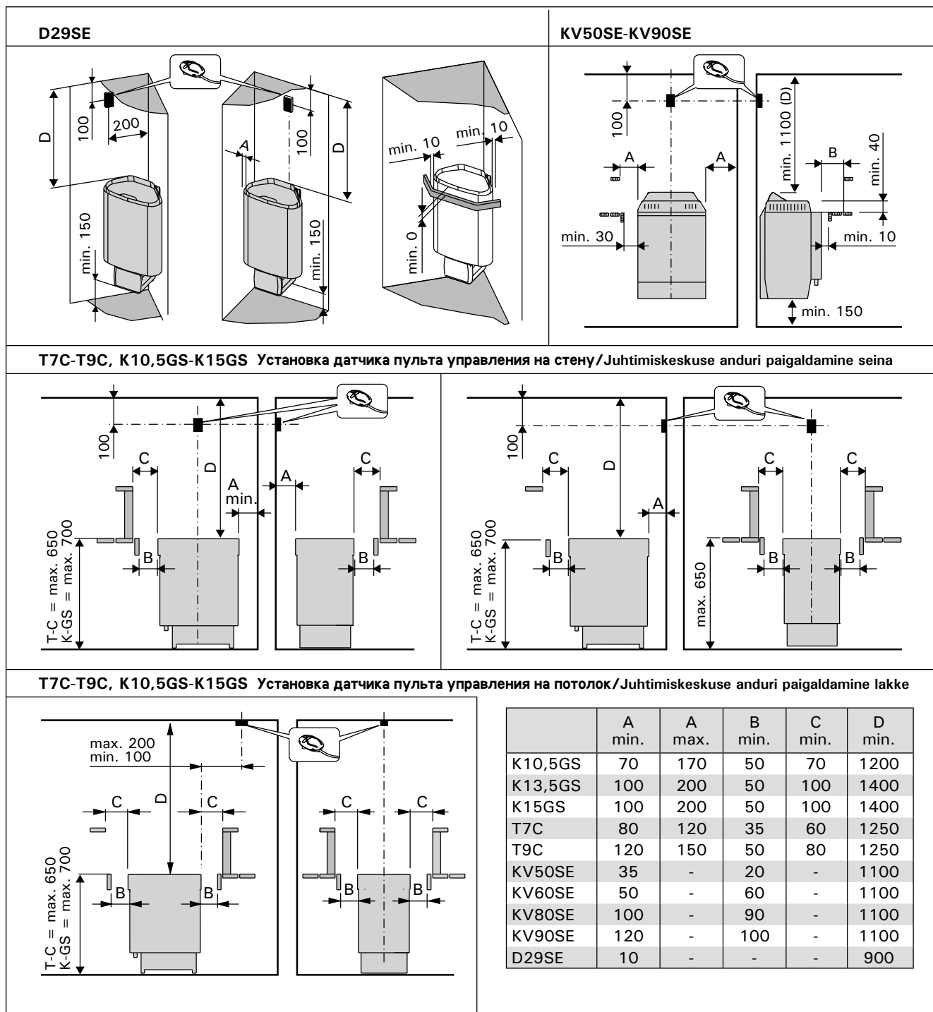
Рисунок 5. Расстояния безопасности (все размеры приведены в миллиметрах) Joonis 5. Kerise ohutuskaugused (kõik mõõtmised millimeetrites)
