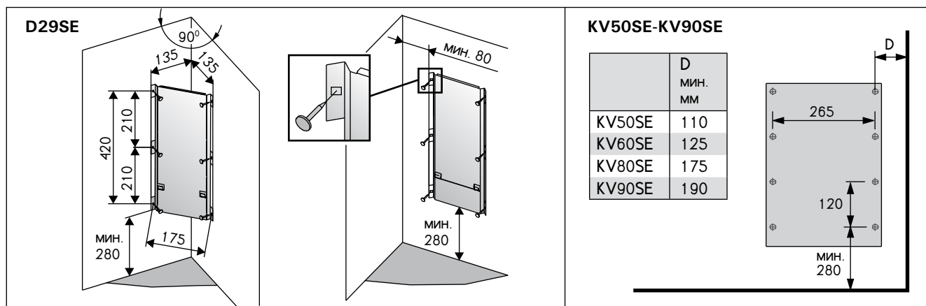
Рисунок 5. Установка крестовой рамы (все размеры приведены в миллиметрах) Joonis 6. Kerise paigaldusraami koht (kõik mõõtmised millimeetrites)
