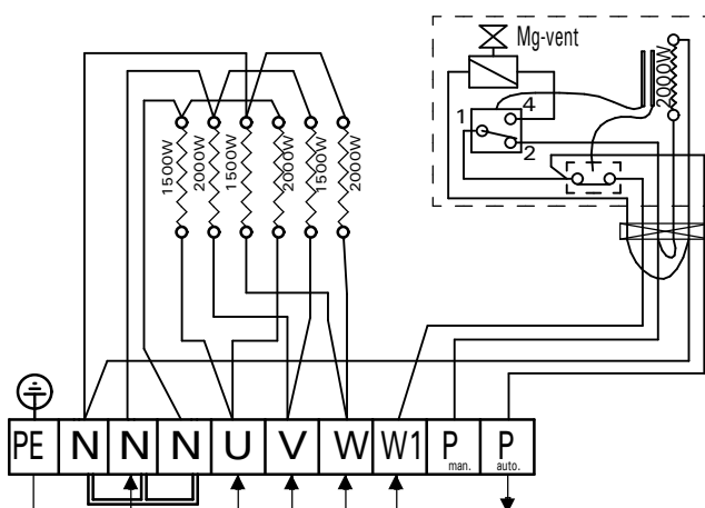
Figure 9. Raccordements électriques Figuur 9. Elektrische aansluitingen
