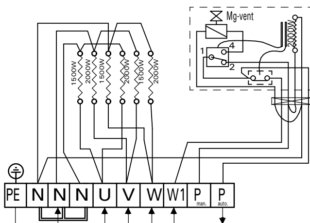
Figura 9. Conexiones eléctricas Figura 9. Collegamenti elettrici
