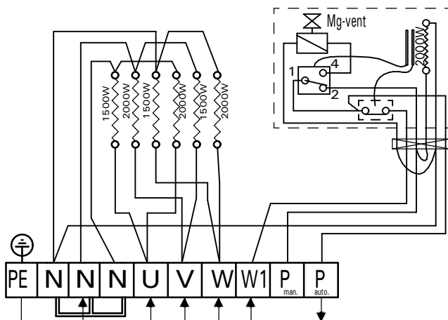
Рисунок 9 Электромонтаж Joonis 9. Elektrihendused
