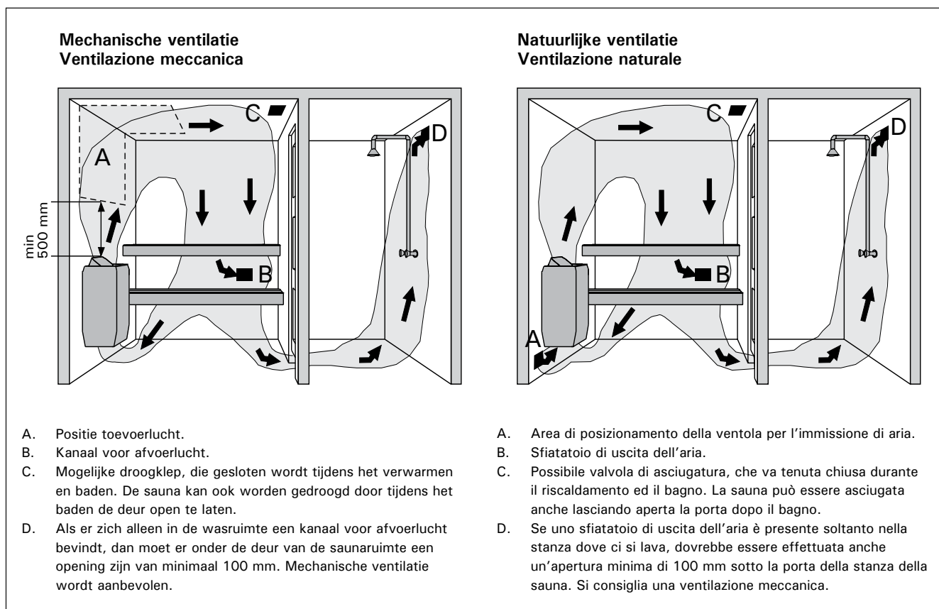
Figuur 7. Ventilatie van de saunaruitte Figura 7. Ventilazione della stanza della sauna
