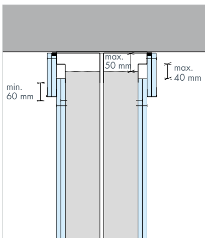
Teleskopskinne TSK-2 DD Max. nedbøjning ved TSK-2 og TSK-2 DD er 40 mm. Brand: EI 60 A2-s1, d0
