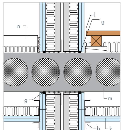
8.6 Tilslutning huldæk på langs
