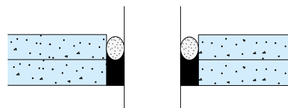
Lydtætning omkring rør og kanaler med fugestopning og fugemasse.
