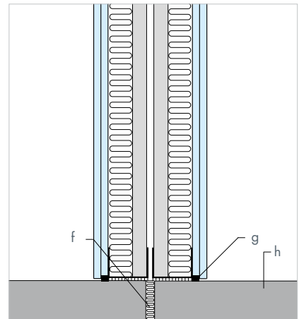
8.3 Tilslutning til massivt gulv
