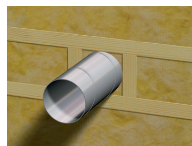
Kubbing rundt gjennomføringer
