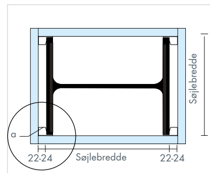
Montage med bjælkeprofil. Søjle.
